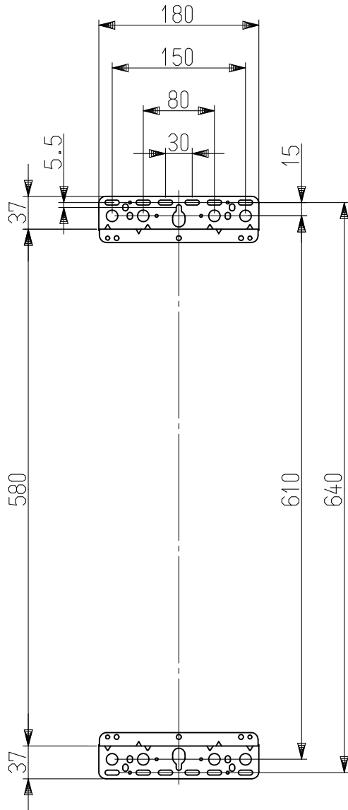
壁掛金具
