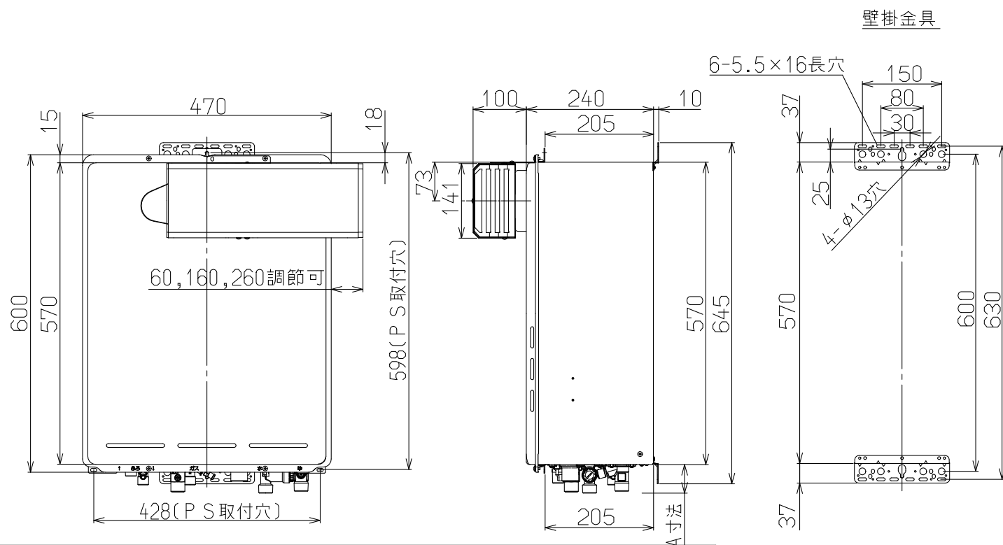
●トリイ配管を行う場合
