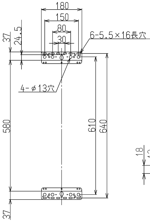
壁掛金具
