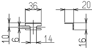
取付金具下(左右共通) 尺度：フリー
