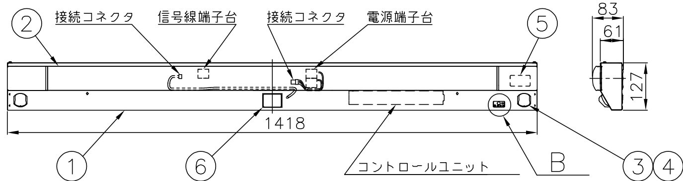
配線図
