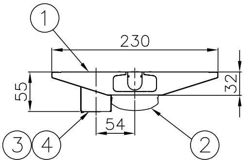
側面詳細図
