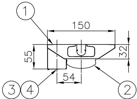
側面詳細図
