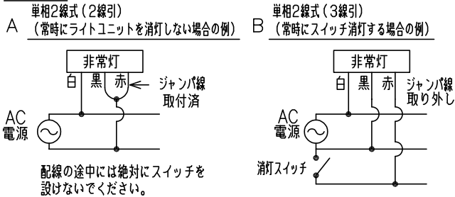
配線図
