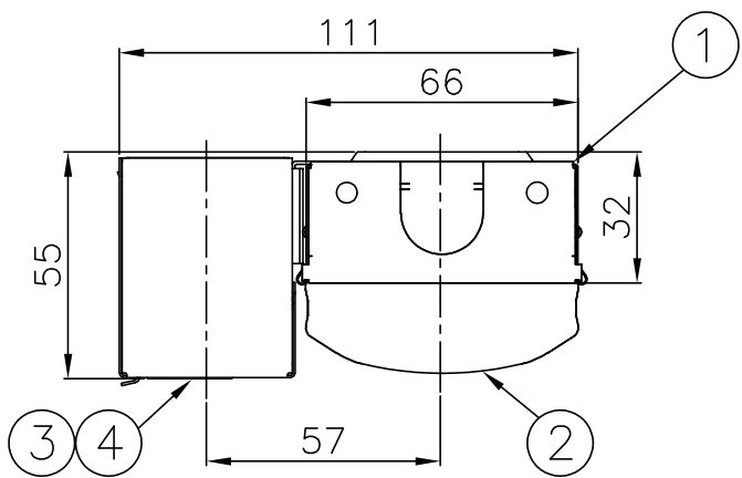
側面詳細図
