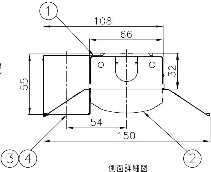
側面詳細図
