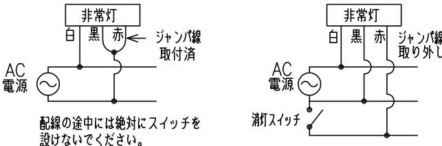
配線図
