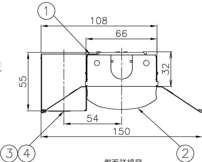
側面詳細図
