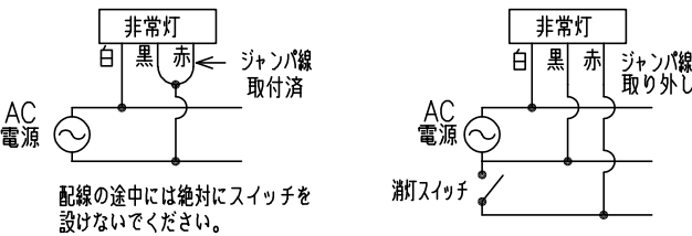
配線図
