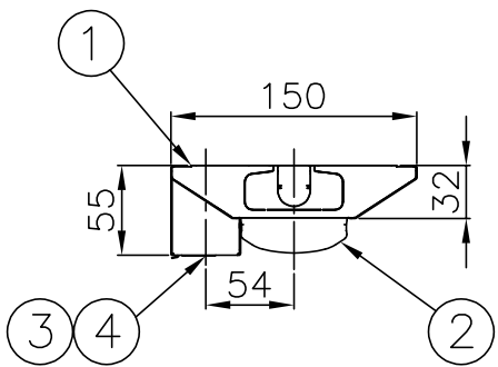
側面詳細図
