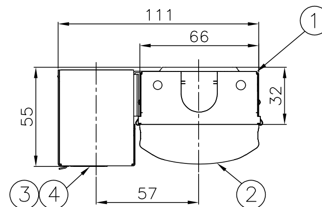
側面詳細図
