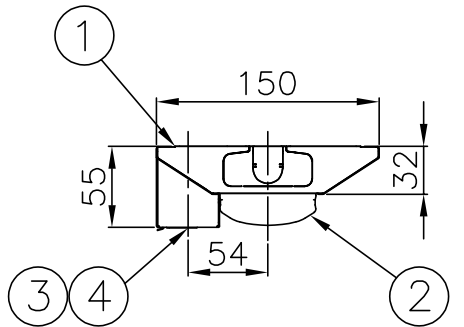
側面詳細図
