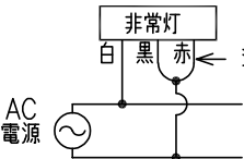
配線図
