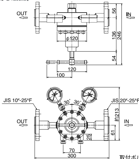
【外観寸法図】
