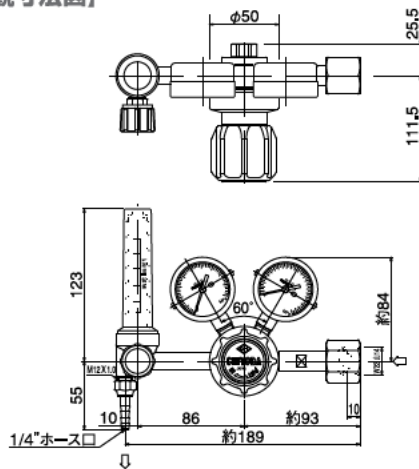
【外観寸法図】
