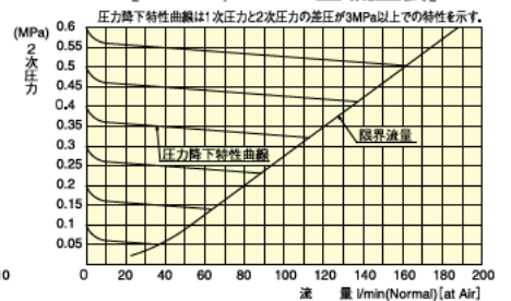
【AHSN-1/AHSN-2型 流量表】
