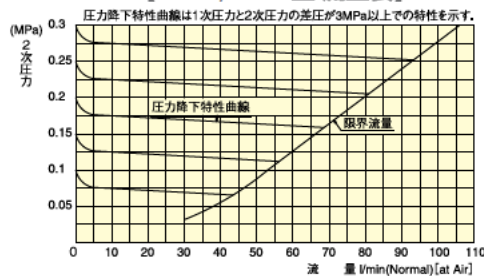
【AHN-1/AHN-2型 流量表】
