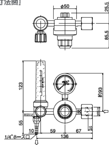
【外観寸法図】
