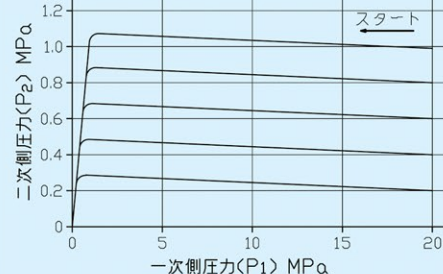
YR-70 圧力変動曲線
