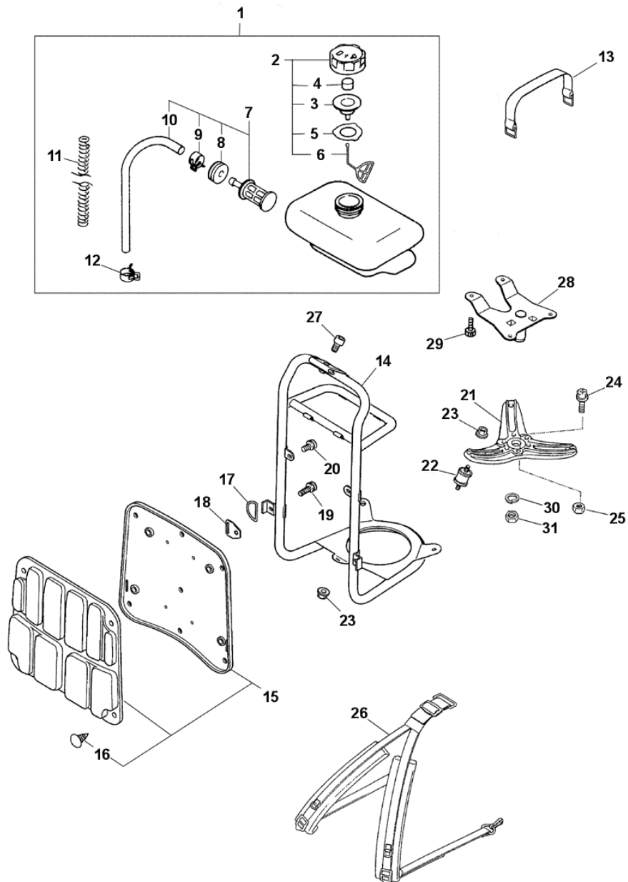
図3 燃料タンク・フレーム
