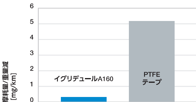
ステンレス製 (SUS303) ピンに対する摩耗データ F = 10N, v = 9,600mm/min
