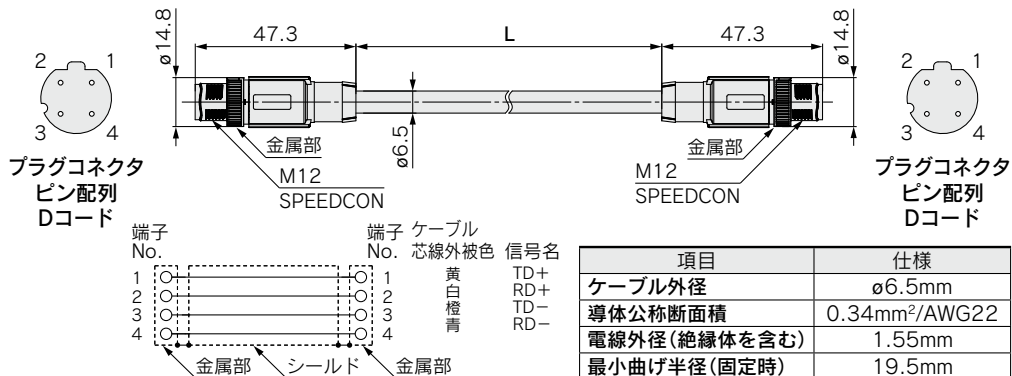
結線図(ストレートケーブル)
