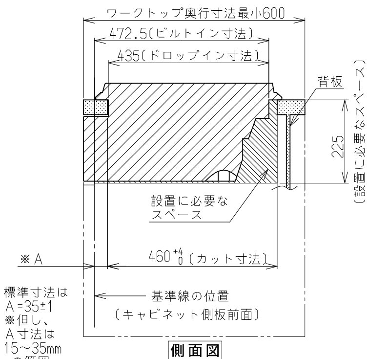
設置施工例図
