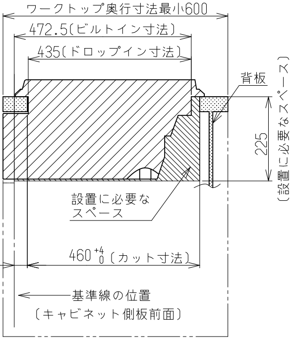
側面図
