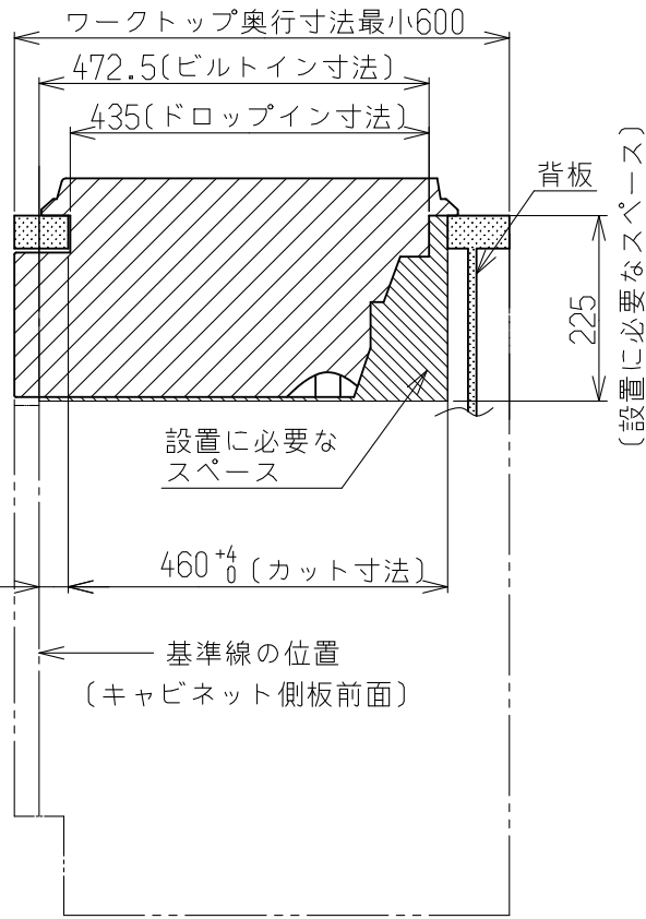
側面図
