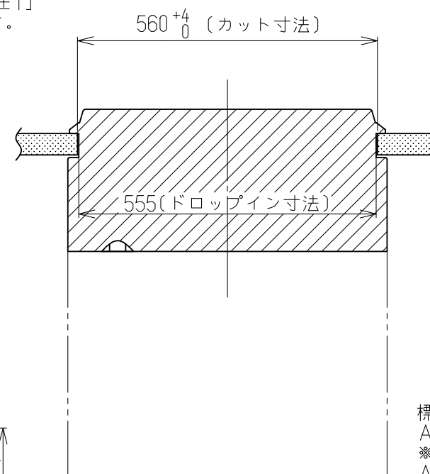
正面図
