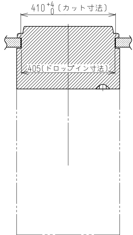
正面図
