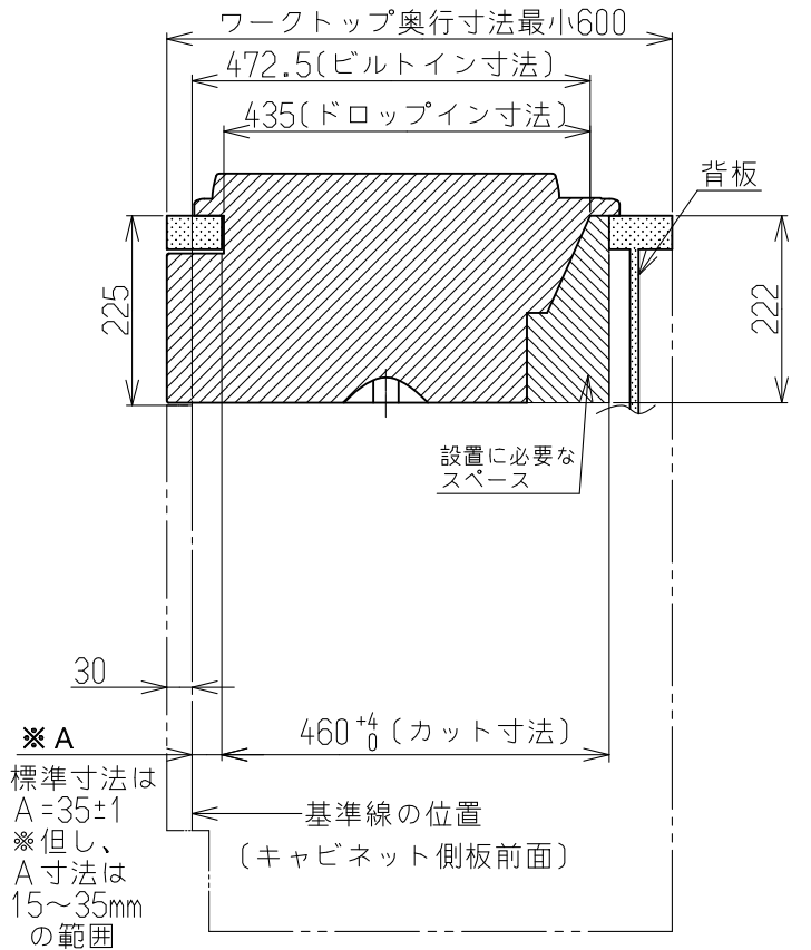
側面図
