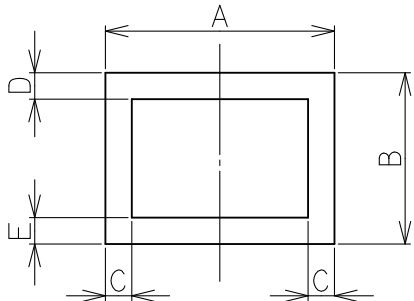
化粧板（パネル材）の寸法（単位mm）
