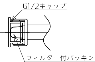
H部拡大図
