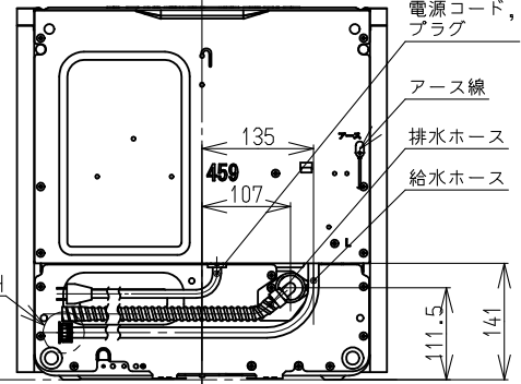
背面図
