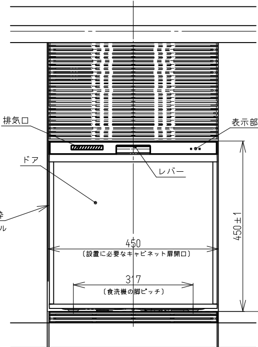
正面図
