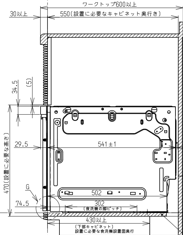
側面図
