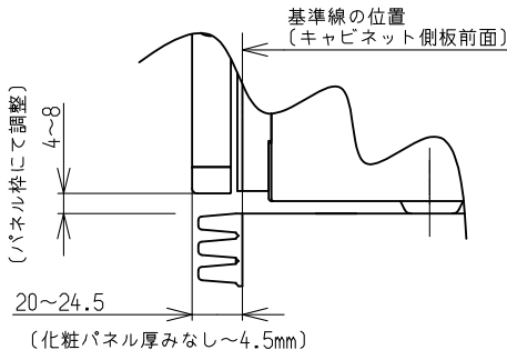
G部拡大図
