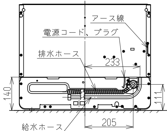
背面図
