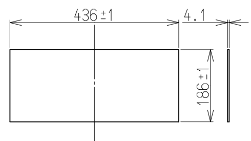
<下パネル材寸法>
