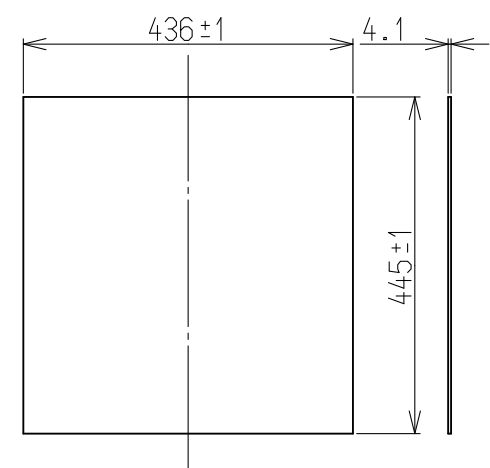
<上パネル材寸法>
