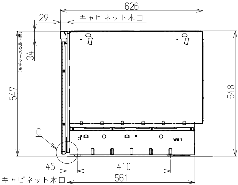
側面図
