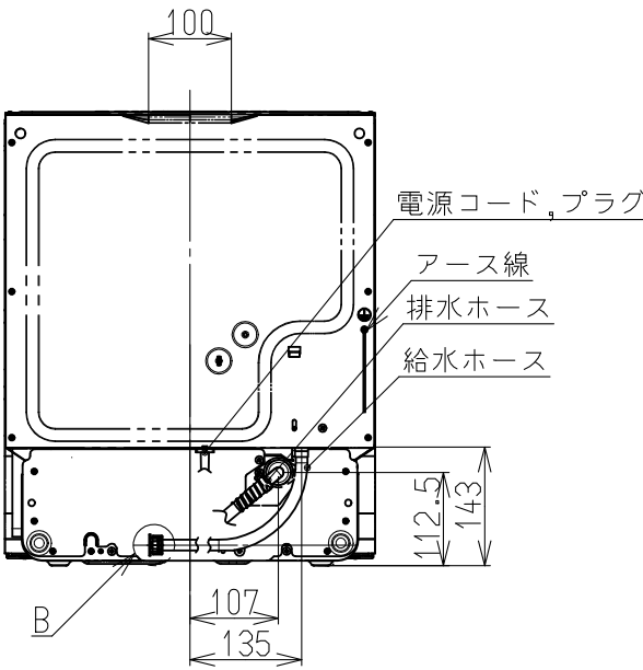
背面図
