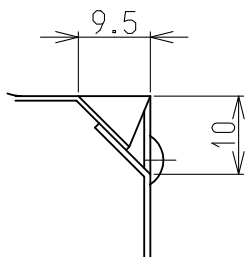
A-A断面拡大図
