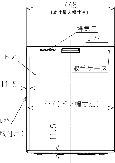
正面図
