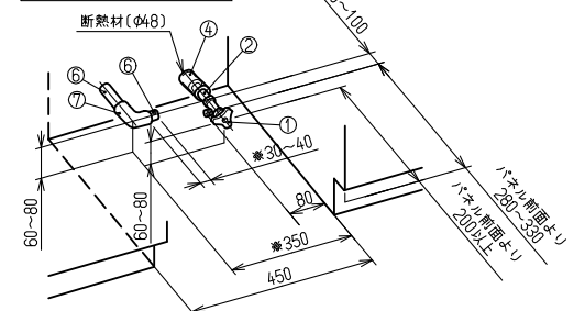
壁出しの配管例
