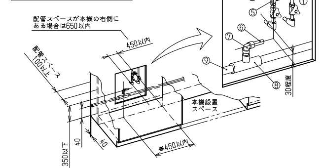
床ころがしの配管例
