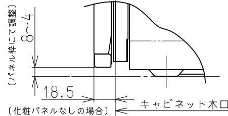
C部拡大図
