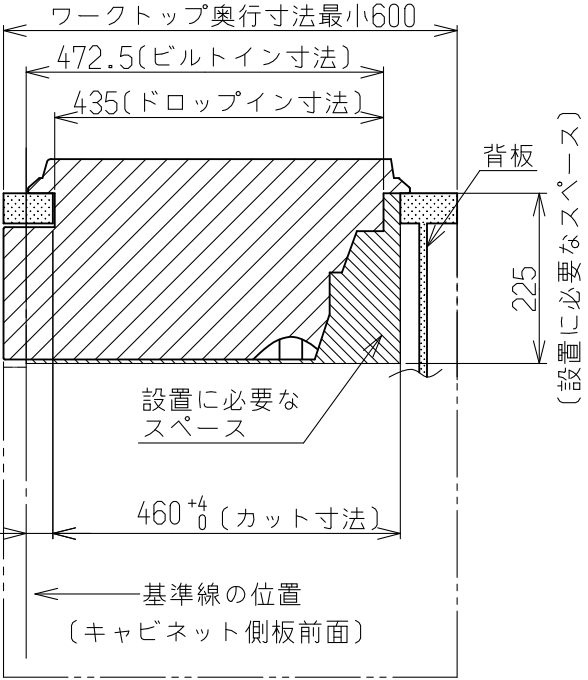
側面図
