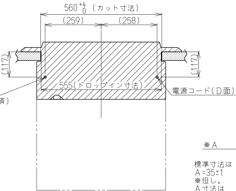
正面図
