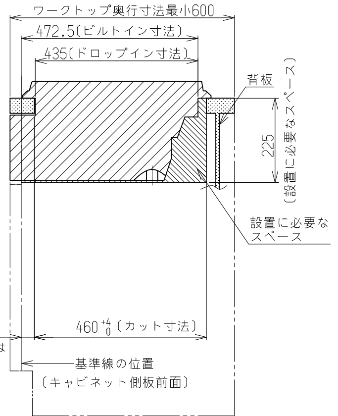
側面図
