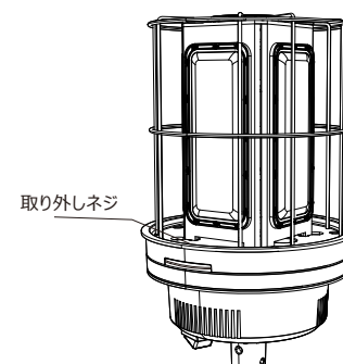
① 取り外しネジを外す
