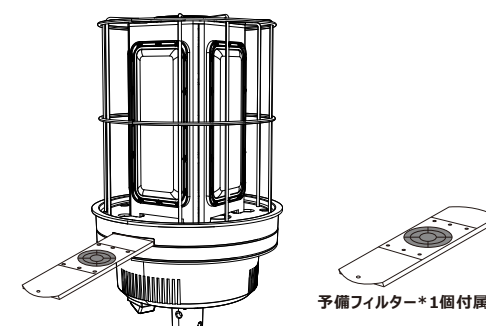
② フィルターを取り出し口から取り出す 取り外したフィルターは水洗い可能です
