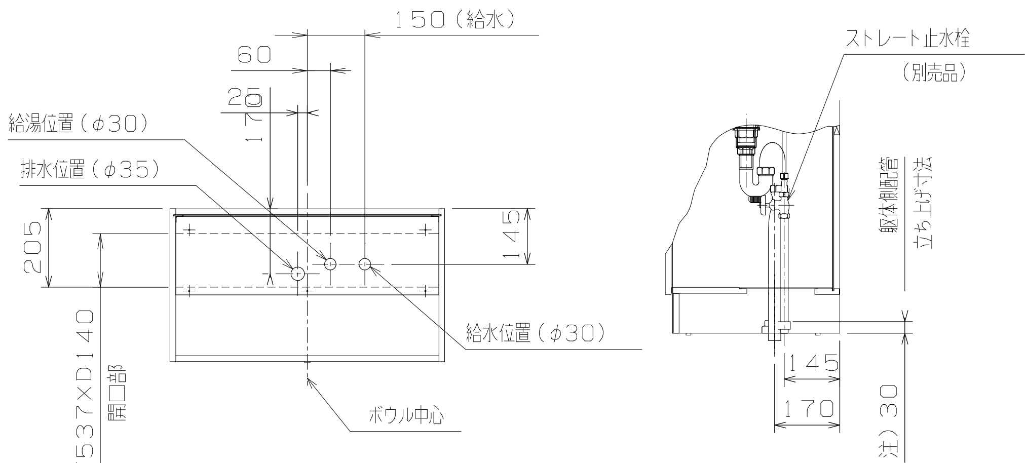
■床給水の場合の配管位置
