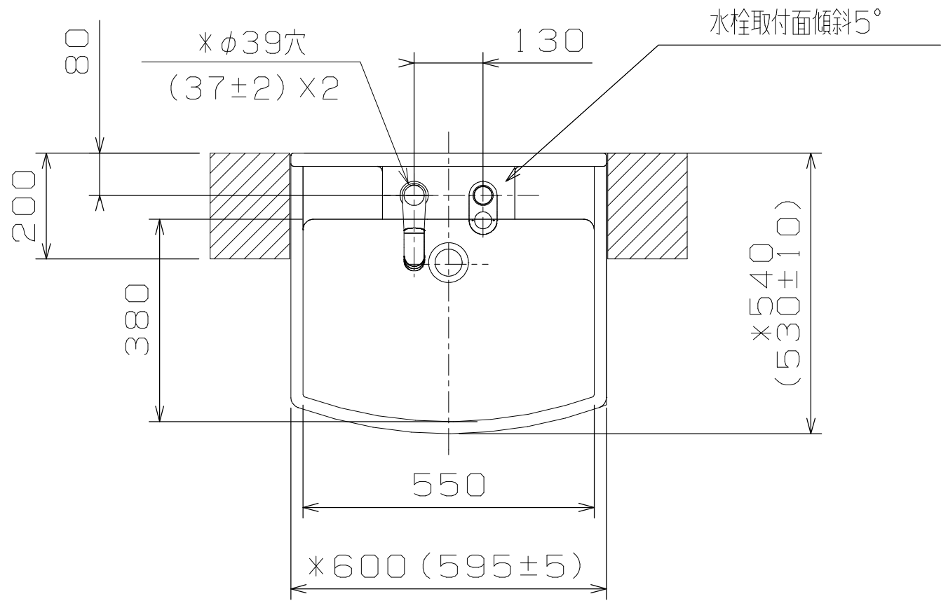
■壁給水の場合の配管位置
