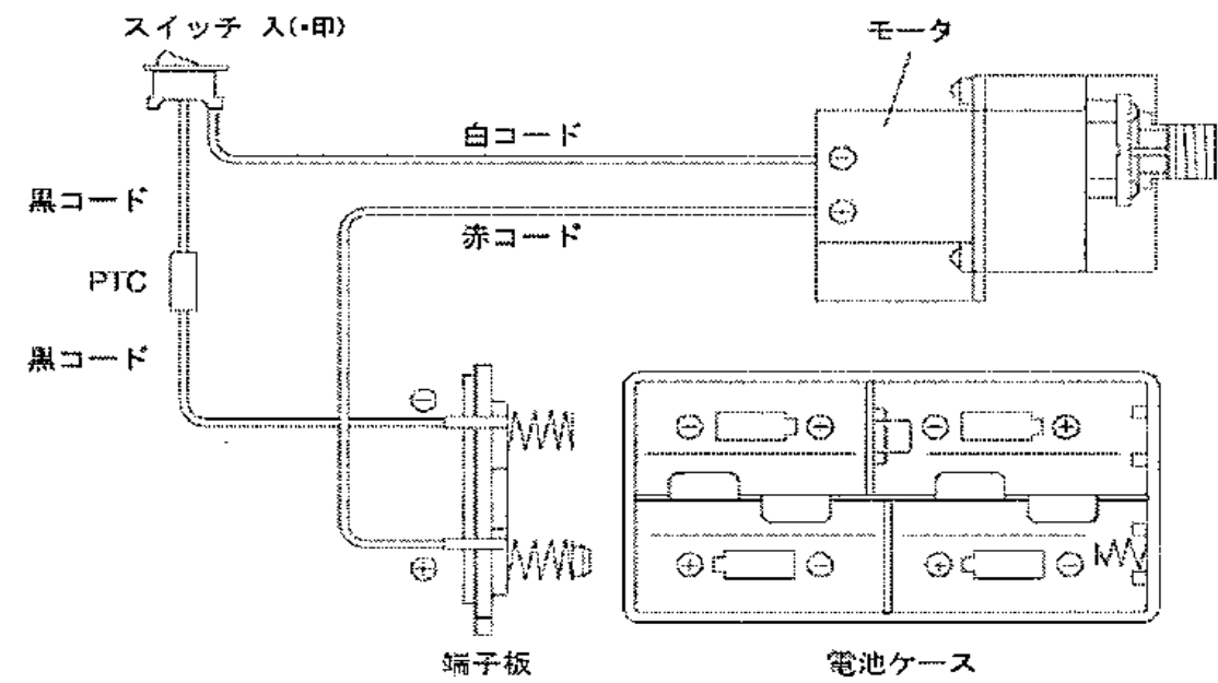
実体配線図
