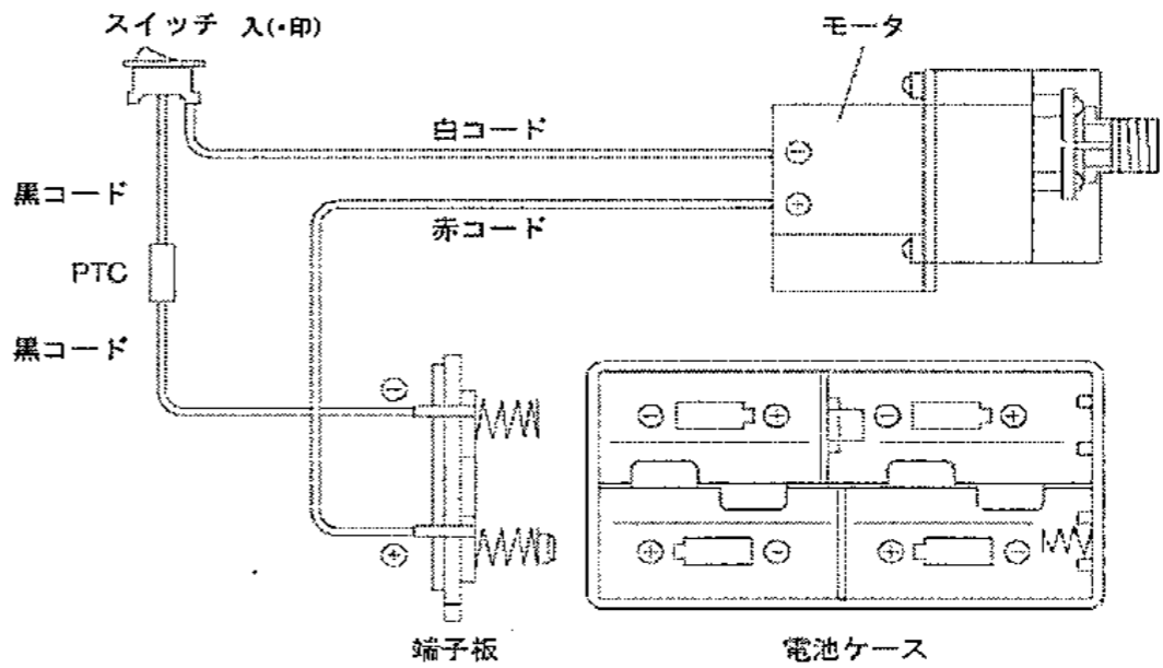
実体配線図
