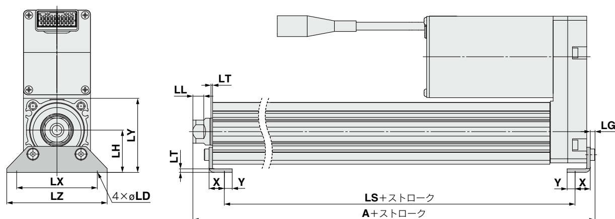
外向き取付の場合
