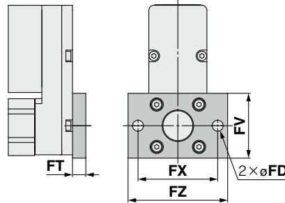
ヘッド側フランジ形/LE2Y 25 / 32 □H A / B -□□□G
