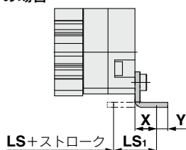
外向き取付の場合
