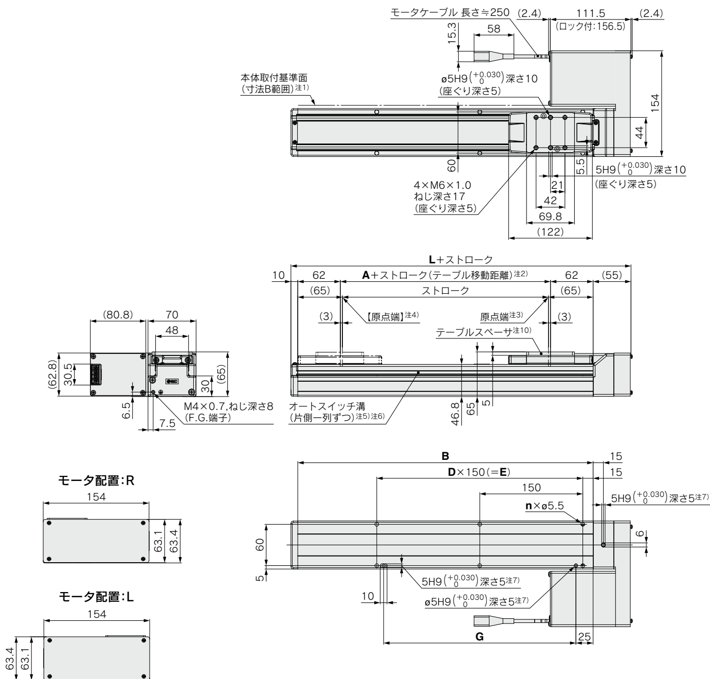
寸法表
