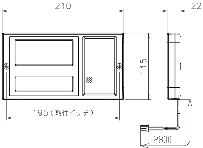
浴室リモコン RC-4024S (尺度1/4)
