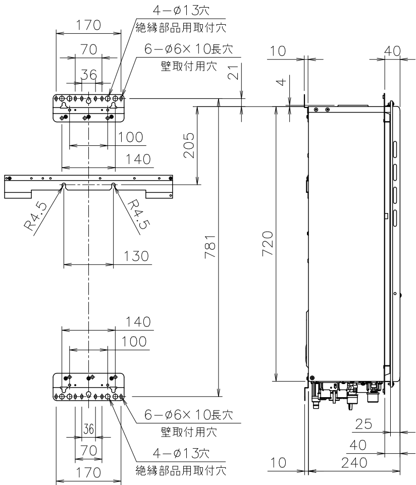
771 (扉内設置用ボックス取付ピッチ)
