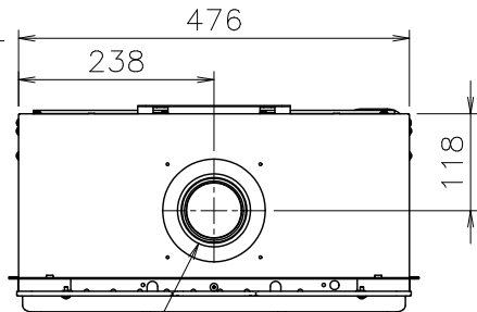
排気接続口φ80
