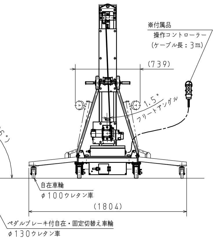
運搬状態
