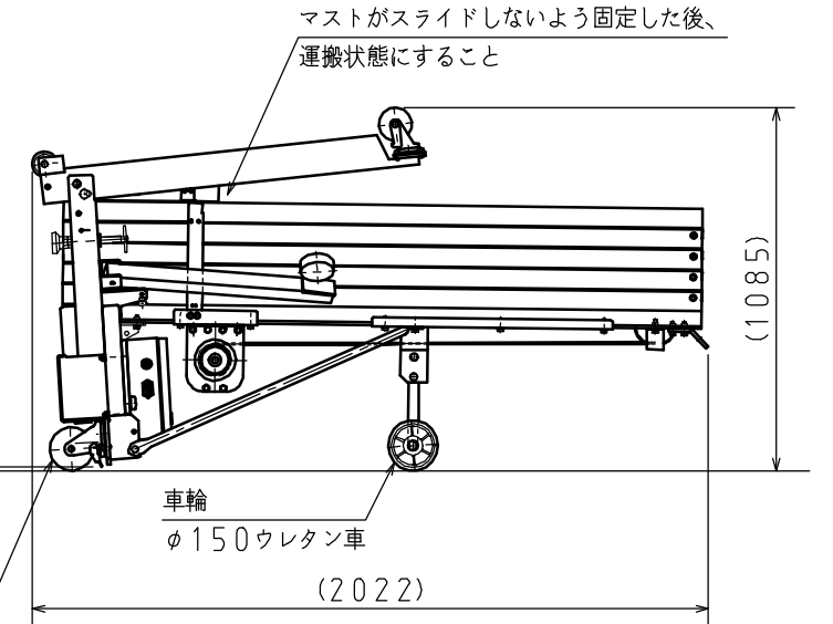
運搬状態
