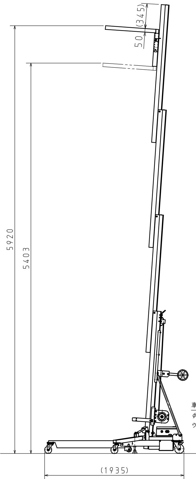
伸長状態 (S = 1 : 30)
