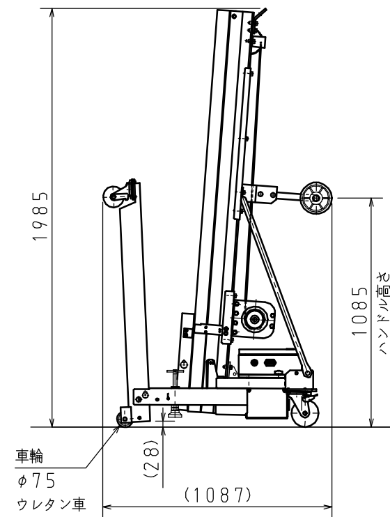
収納状態
