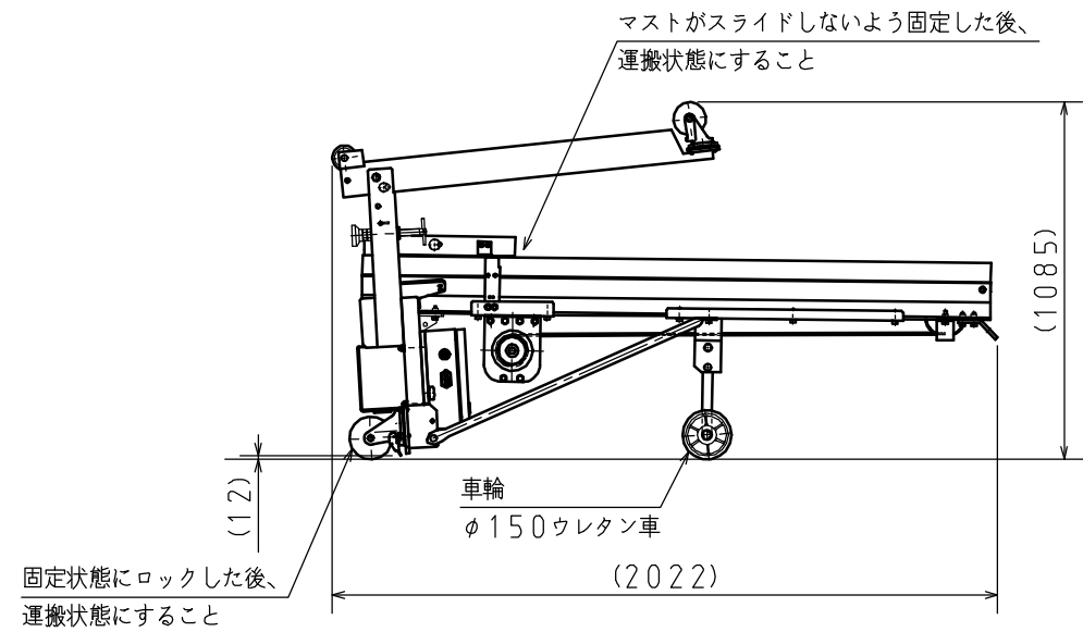
運搬状態
