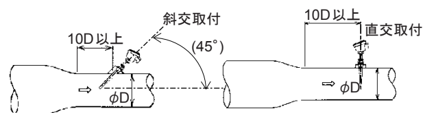
図4 ねじ接続：絞り管路のある管への設置
