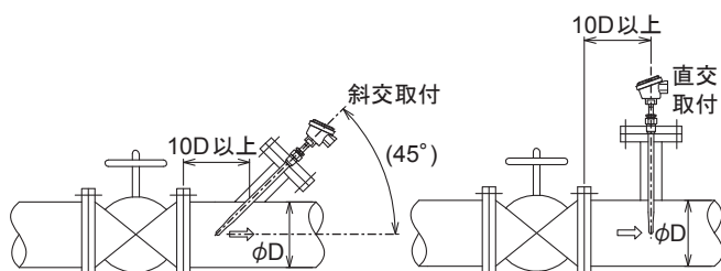
図10 フランジ接続：他の設置機器があるときの設置
