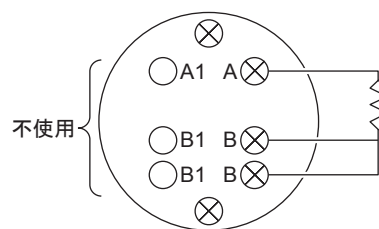
図13 結線図（シングルエレメント）
