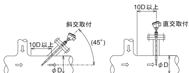
図8 フランジ接続：T継手+ストレート管設置
