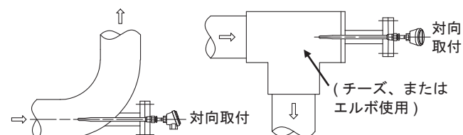
図11 フランジ接続：曲がり管設置 10D以下
