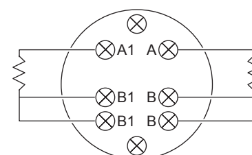
図14 結線図（ダブルエレメント）
