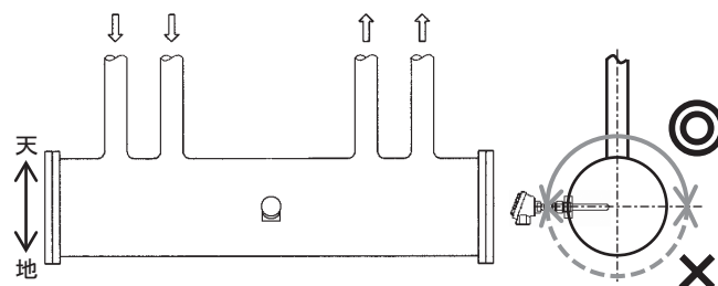
図12 ヘッダーへの設置
