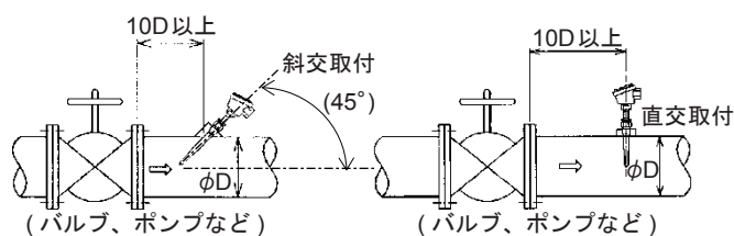
図5 ねじ接続：他の設置機器があるときの設置
