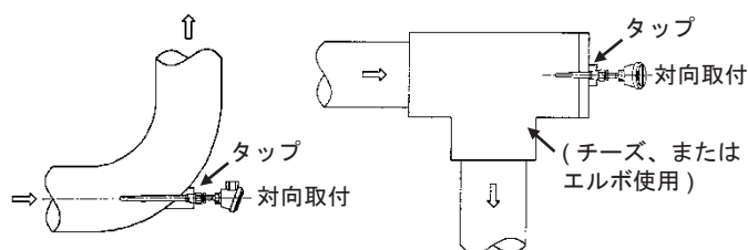
図6 ねじ接続：曲がり管設置 10D以下
