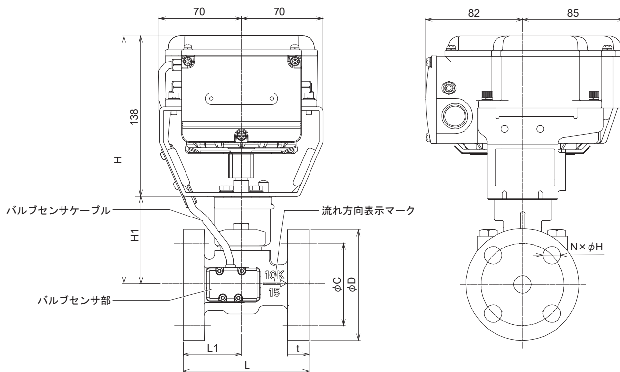
図2 外形寸法図 (mm)
