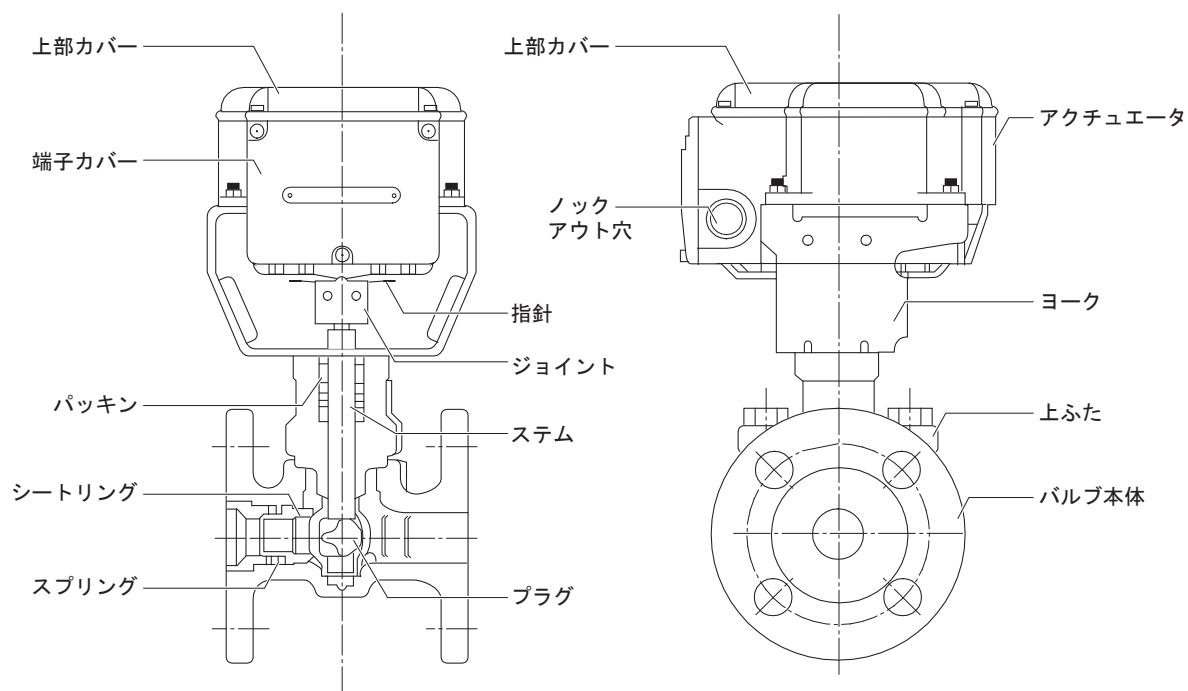
図4 各部の名称
