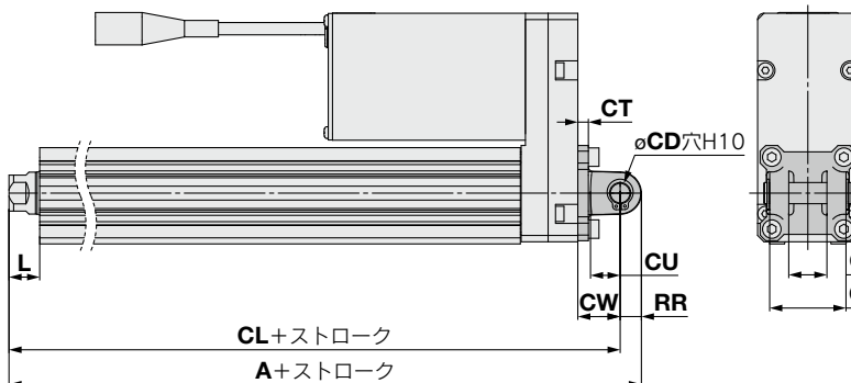
2山クレビス形/LE2Y 25 32 □H A B -□□□D H A B C
