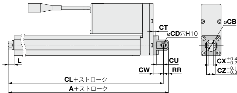
2山クレビス形/LE2Y 25 32 □H A B -□□□D H A B C
