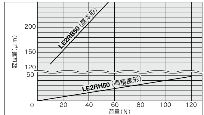
LE2R□50
