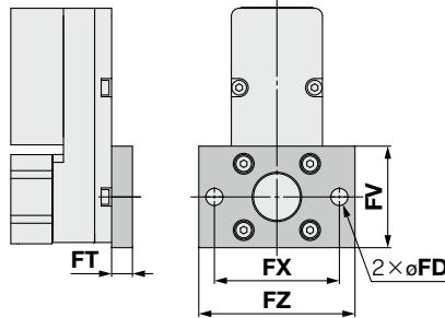
ヘッド側フランジ形/LE2Y 25 32 □H A B -□□□G H A B C
