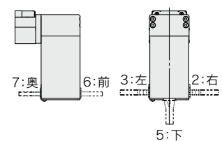
モータ配置:U ケーブル取出し図
