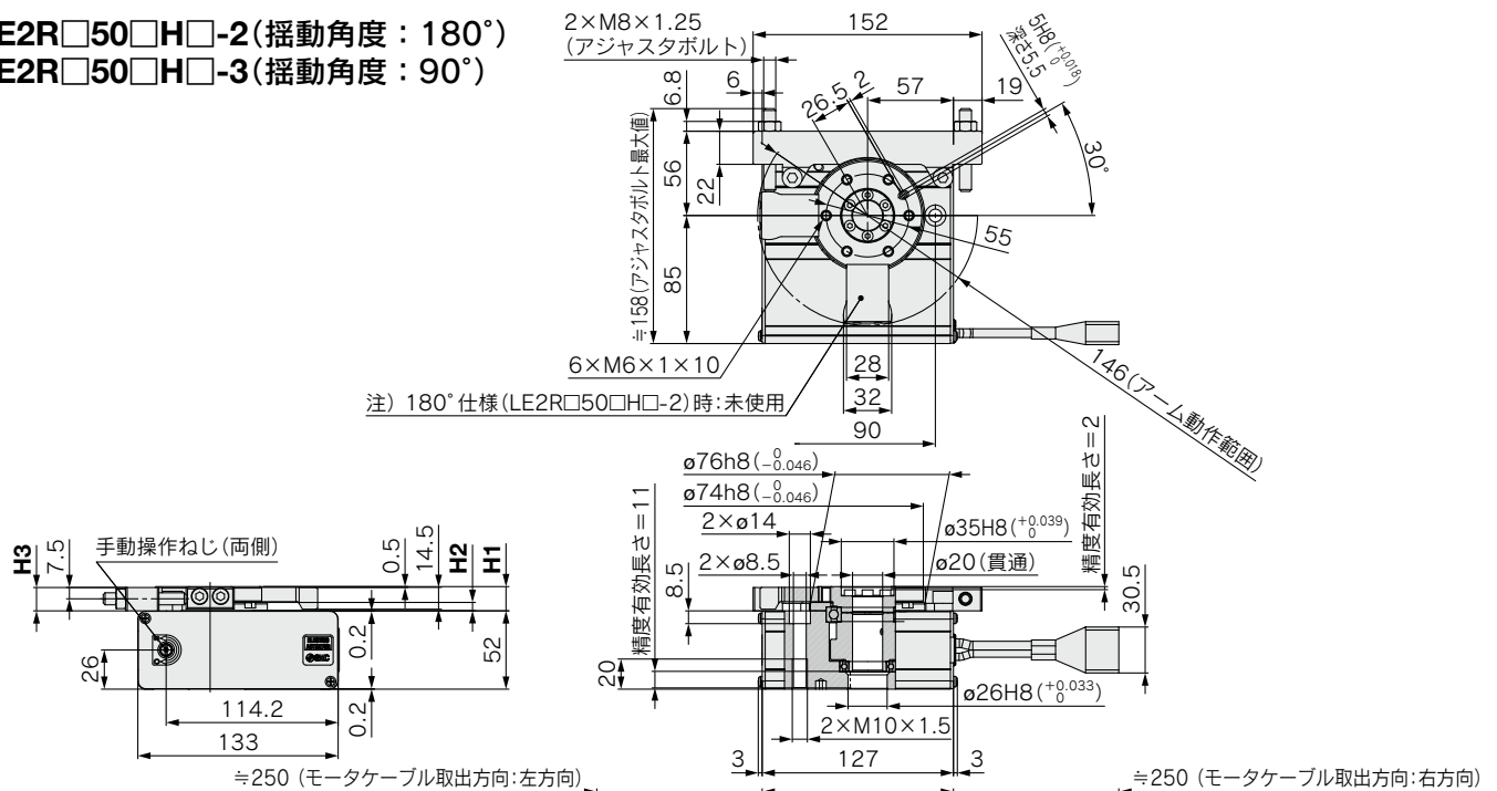
寸法表 [mm]
