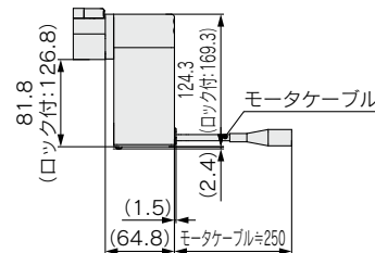
モータ配置:U
