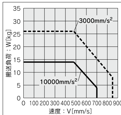
〈速度-搬送質量グラフ〉 (LE2FS25H/バッテリレス アプソ)
