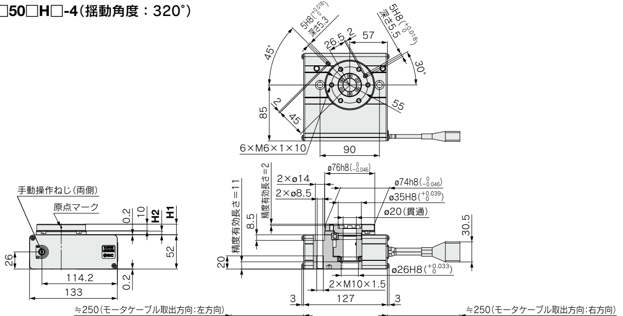
寸法表 [mm]
