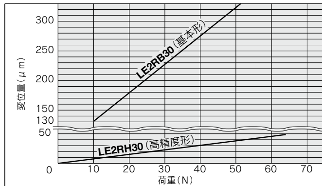
LE2R□30
