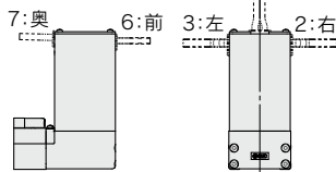
モータ配置:T ケーブル取出し図
