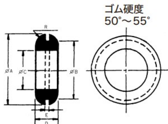
B型 (TO-572)
