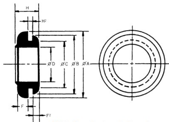
膜付グロメット (TO-584)
