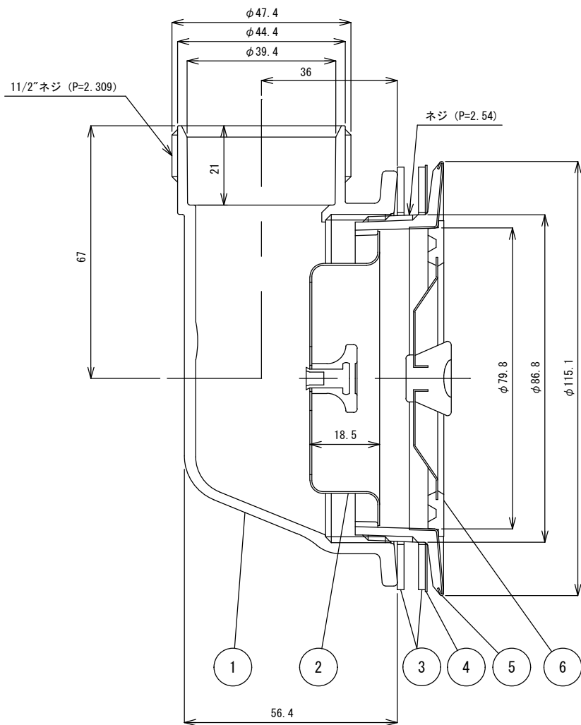
A-A' 断面
