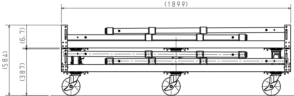
折りたたみ積み重ね詳細図
