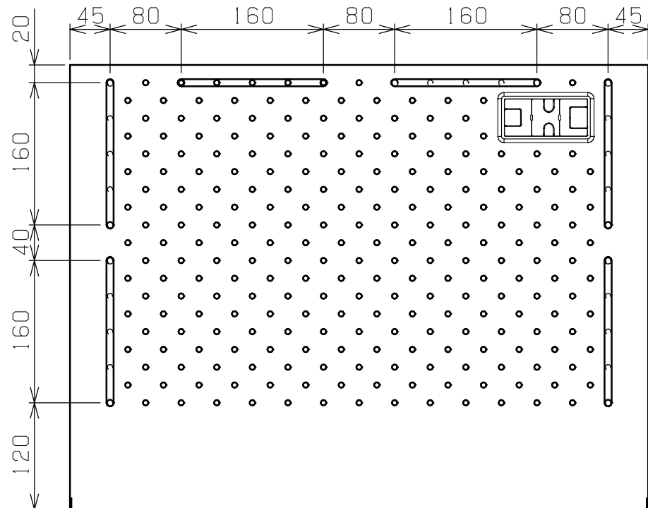
オプションコボレ止め3セット取り付け（天棚の場合）
