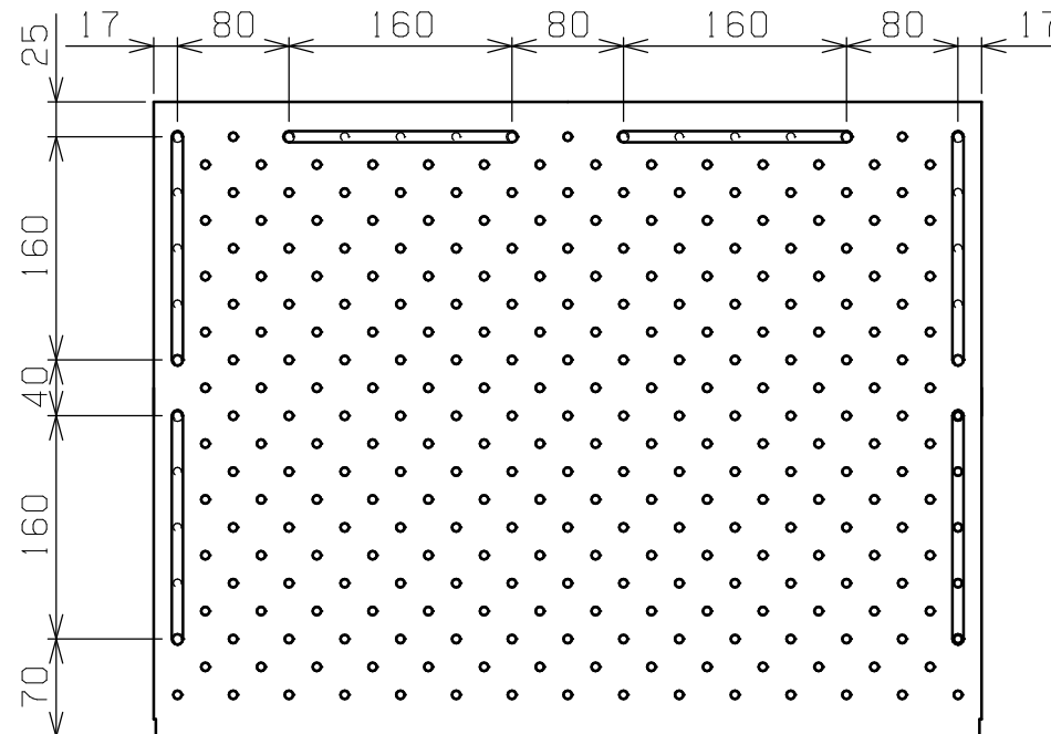
オプションコボレ止め3セット取り付け（中棚の場合）
